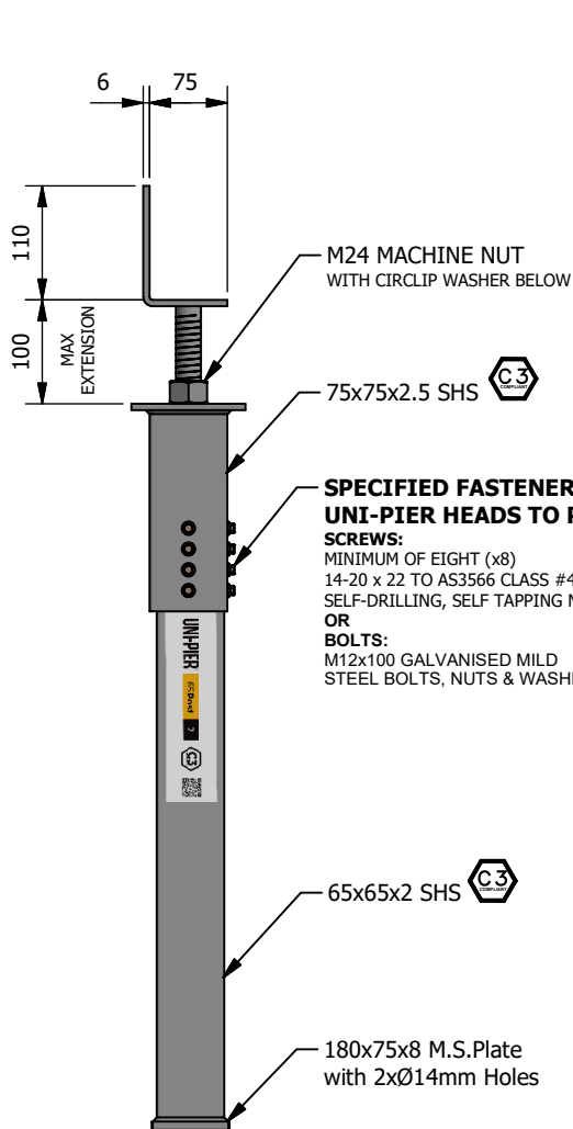
ELEVATION 2
