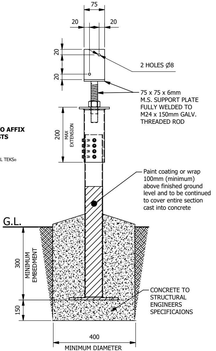
ELEVATION 1
