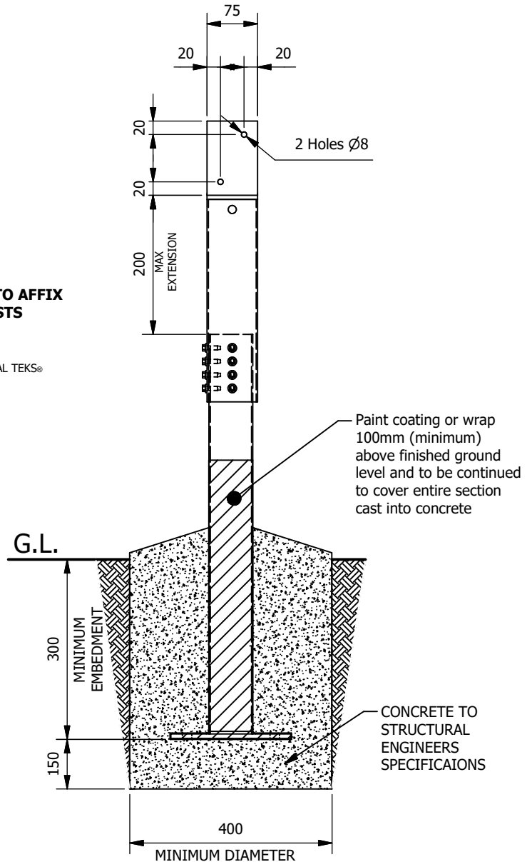
ELEVATION 1
