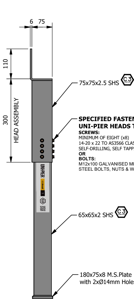
ELEVATION 2
