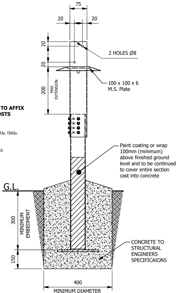
ELEVATION 1
