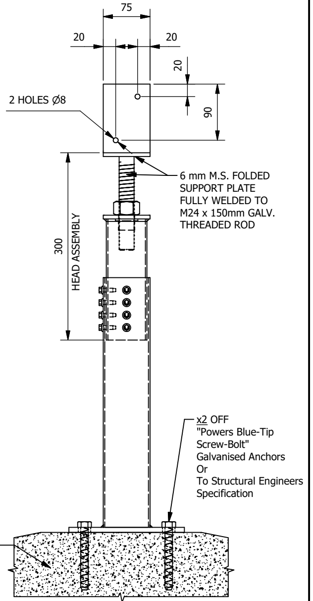
ELEVATION 1
