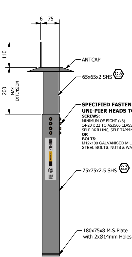
ELEVATION 2
