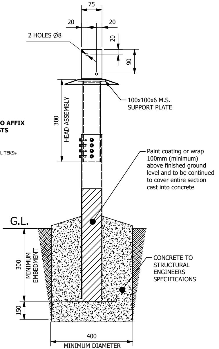
ELEVATION 1
